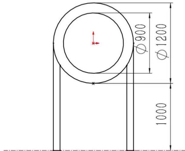
图 6 圆环示意图
