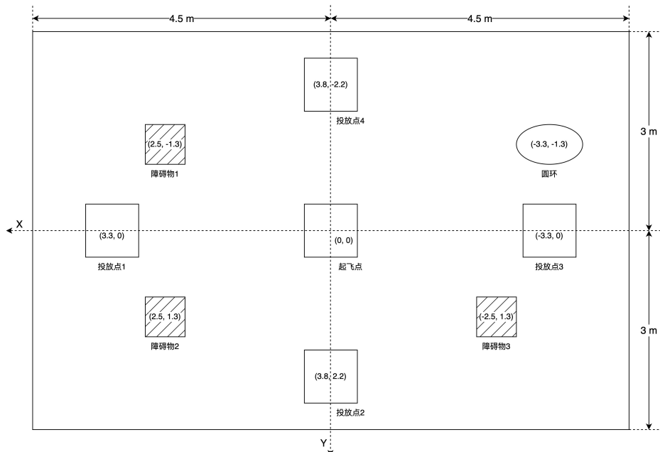
图 2 场地示意图
